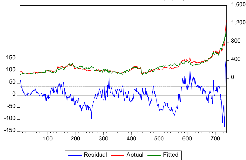
Fig 17. Actual vs. Predicted
