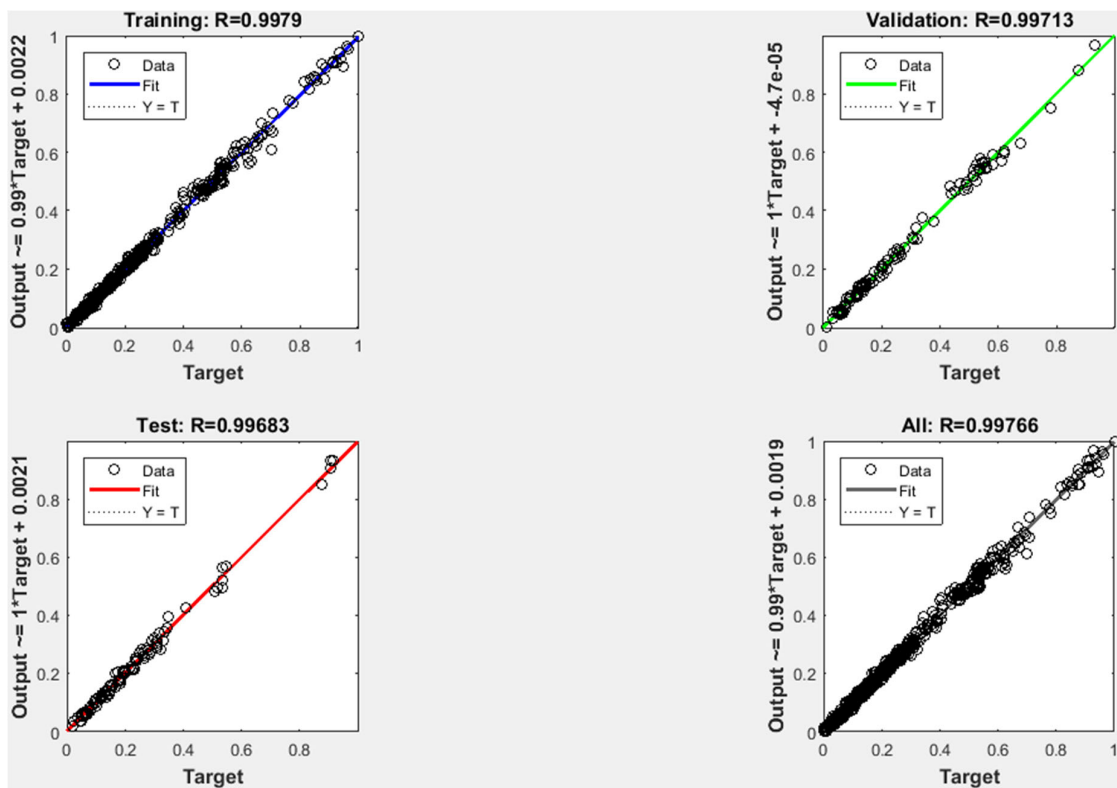
Fig. 11. ANN Regression
